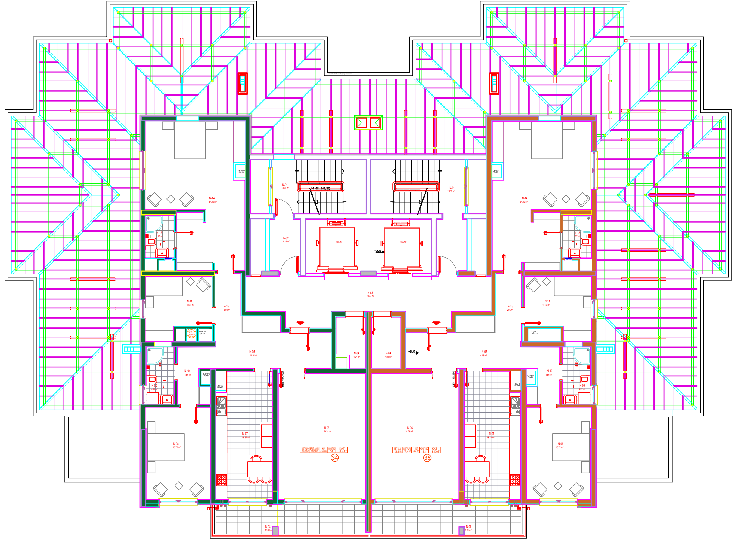
ANKARA SINCAN SARAYCIK MAHALLESİ G.Ö.B. KENTSEL DÖNÜŞÜM PROJESİ SA TİP BLOK 8. KAT PLANI
