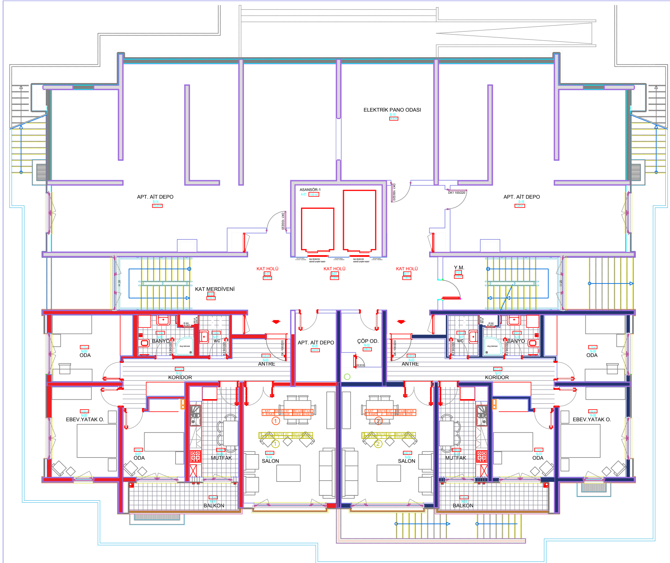
ANKARA SINCAN SARAYCIK MAHALLESİ G.Ö.B. KENTSEL DÖNÜŞÜM PROJESİ SC2 TİP BLOK BODRUM KAT PLANI
