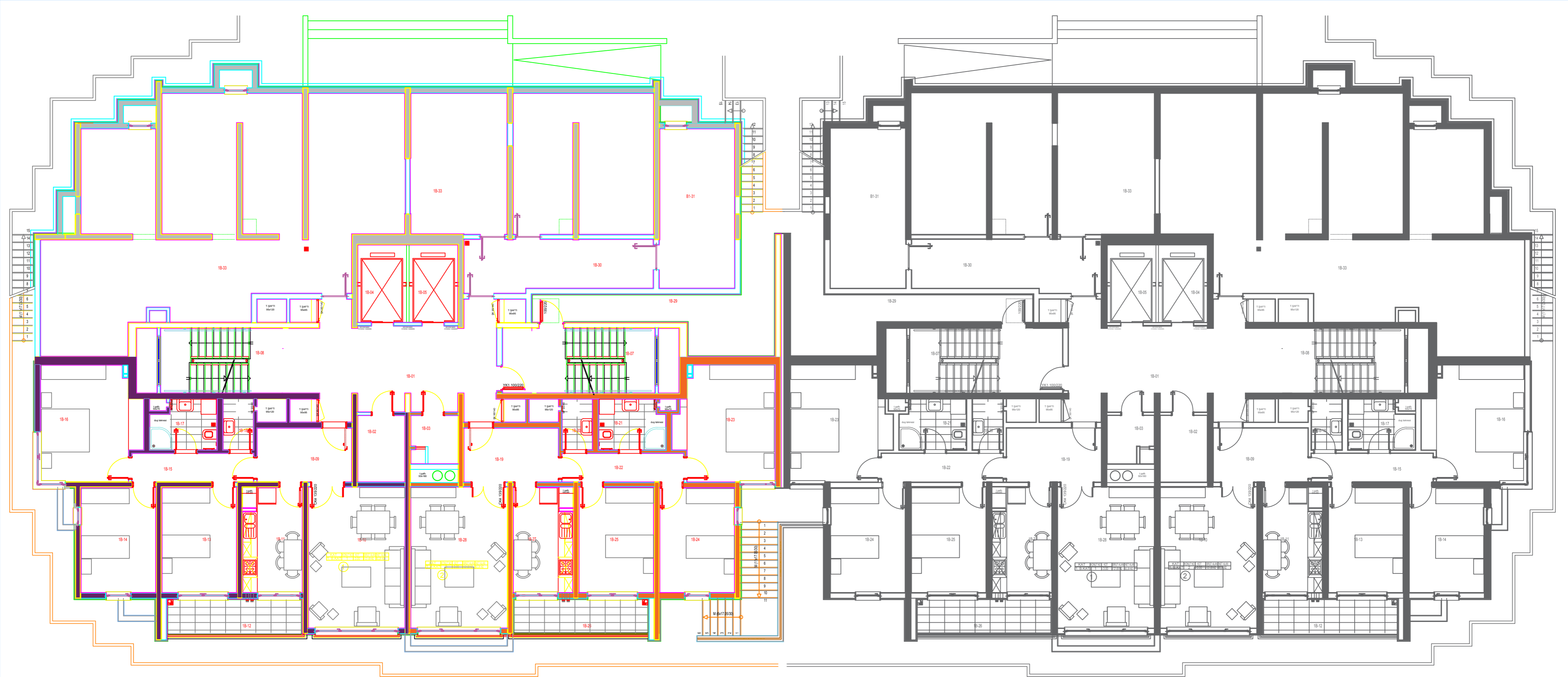
ANKARA SINCAN SARAYCIK MAHALLESİ G.Ö.B. KENTSEL DÖNÜŞÜM PROJESİ SC3 TİP BLOK BODRUM KAT PLANI
