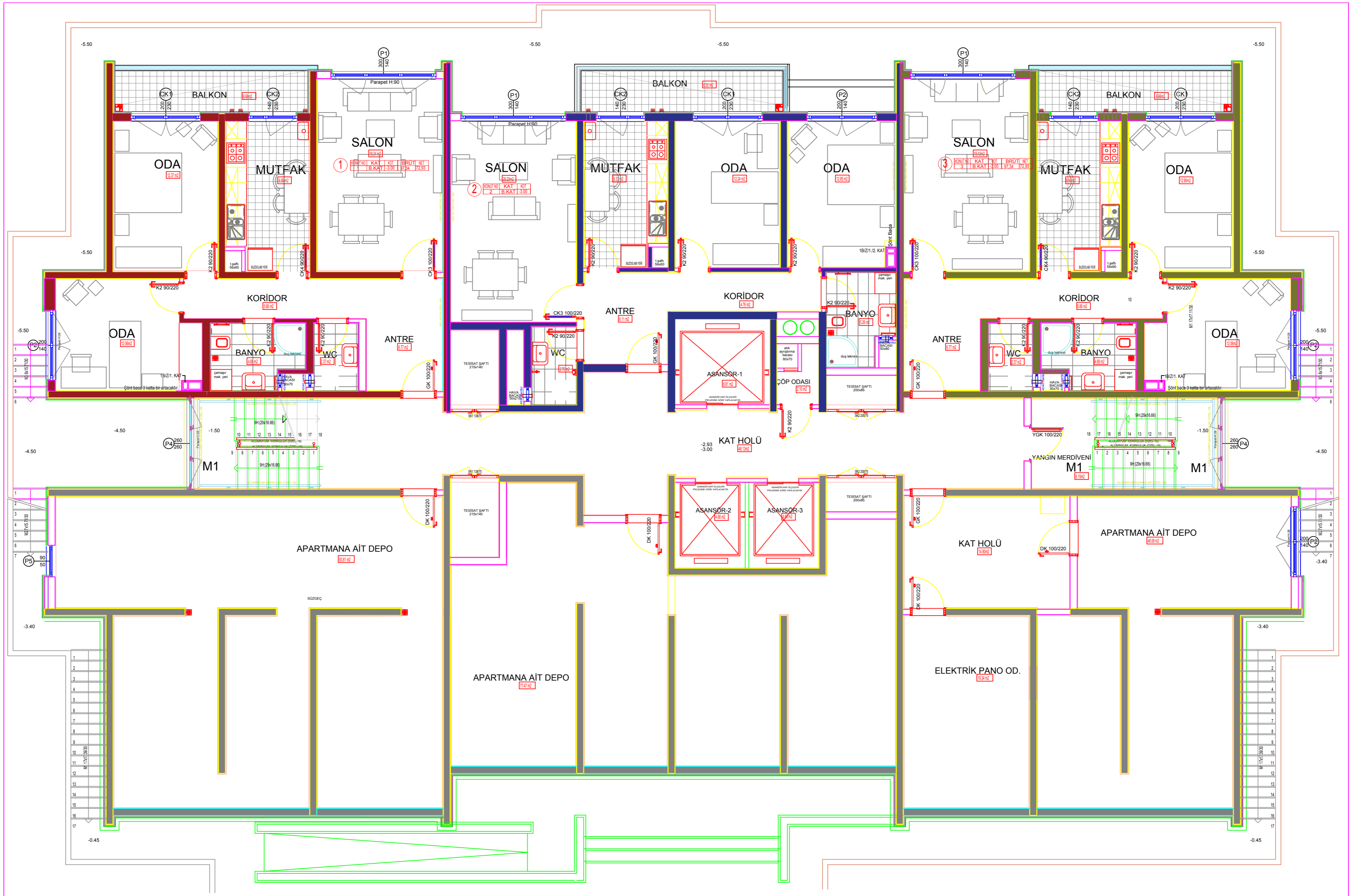
ANKARA SINCAN SARAYCIK MAHALLESİ G.Ö.B. KENTSEL DÖNÜŞÜM PROJESİ SF TİP BLOK BODRUM KAT PLANI
